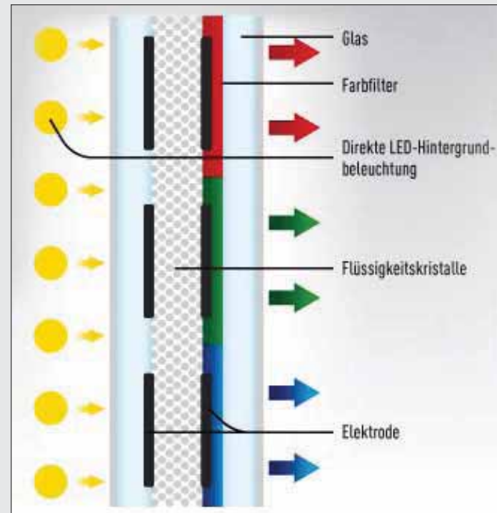
Aufbau eines einzelnen LCD-Pixels (Quelle: http://img2.hifi-regler.biz/pictures/special/direct-led-technologie.jpg )
